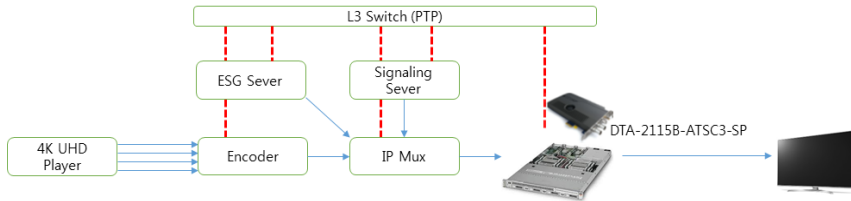
〈연구용 UHD Head-End 시스템 구성도〉
